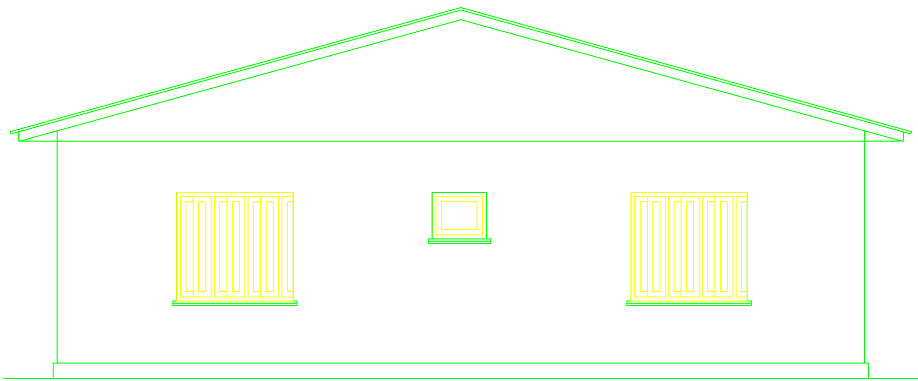
FACHADA LESTE ESC. 1:50
